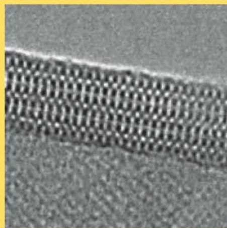
H-9500 300kV x300k 10nm
